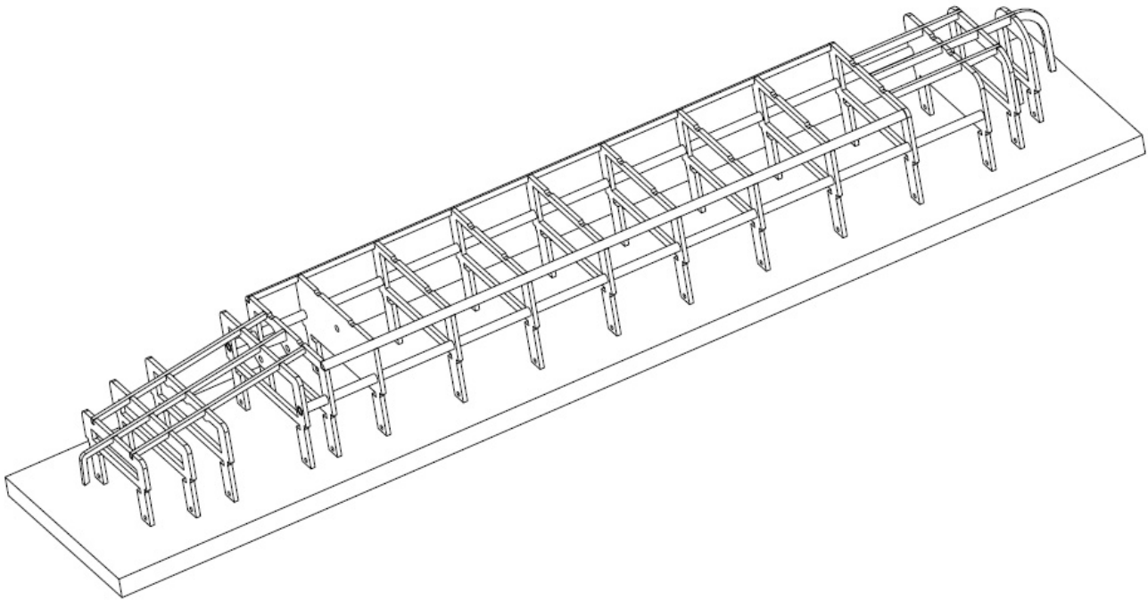
Das Spantgerüst
